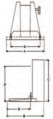
機械尺寸 (Machine Dimensions)
