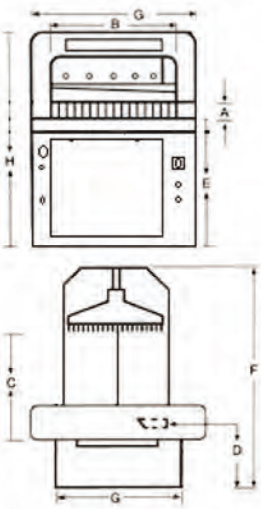
機械尺寸 (Machine Dimensions)
